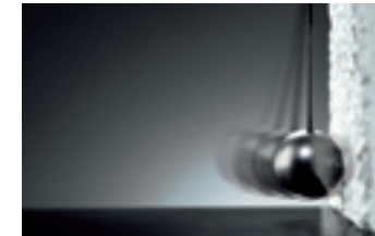
Pendelschlagversuch mit 4 Joule Belastung
